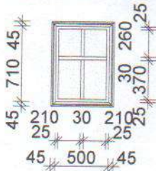
Вікно М 1:50
