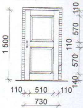
Двері М 1:50
