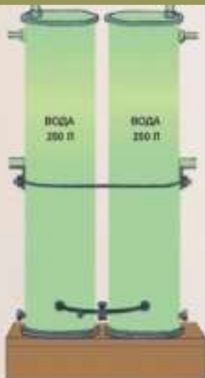
Вертикальний бак аварійного запасу води
